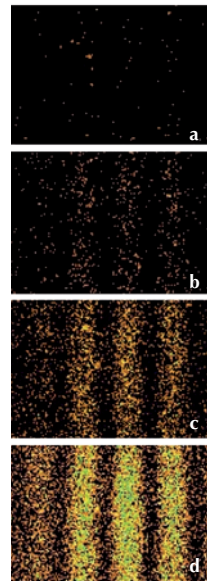
7 ▶ Construction de franges d'interférences photon par photon. En (a), les photons se présentent un par un, ce qui est typique d'un comportement corpusculaire. En (b), (c) et (d), l'accumulation d'un grand nombre de photons fait apparaître une figure d'interférences, preuve indiscutable de la nature ondulatoire de la lumière (Thèse V. Jacques 2007)
