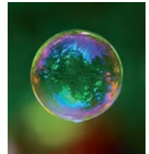
4 ▶ Les interférences sont à l'origine des couleurs irisées d'une bulle de savon. En haut, le dispositif des fentes de Young permet de mettre en évidence les interférences entre deux ondes de lumière. © iStock.com/Jeff Kubina et Daniel Hennequin
