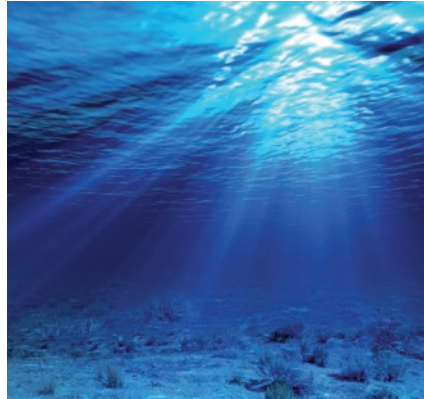
2 ▶ Observation naturelle de trajectoires rectilignes de la lumière. © iStock.com/RomoloTavani
